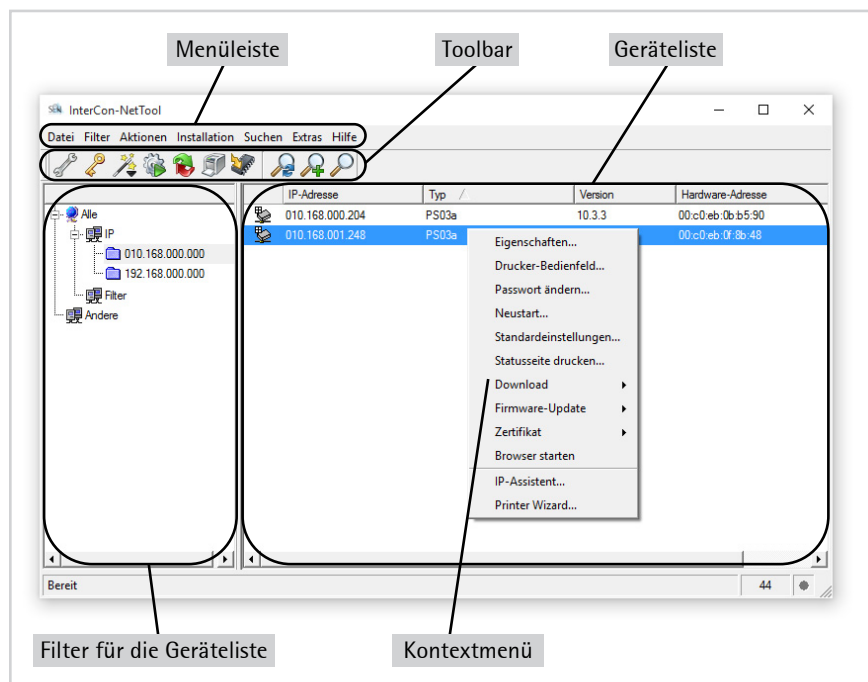
Abb. 2: InterCon-NetTool - Hauptdialog
