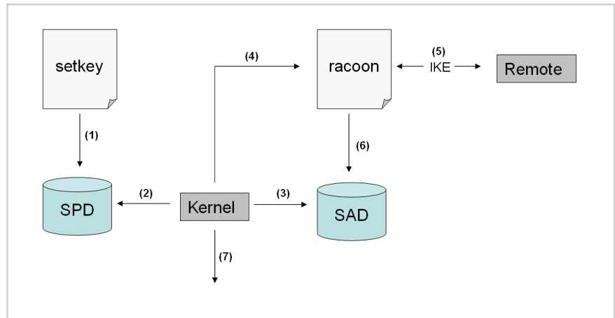
Abb. 9: IPsec-Ablauf
